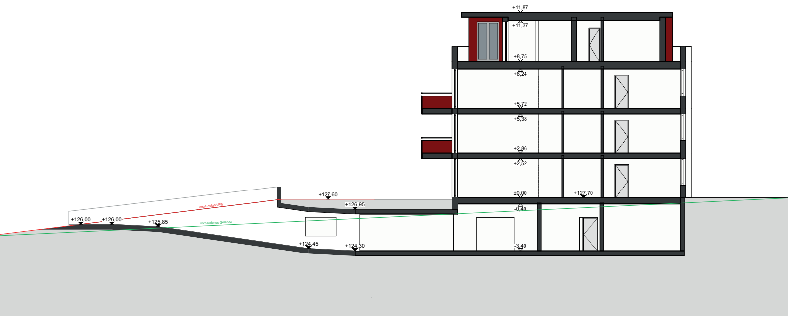
SCHNITT B-B
